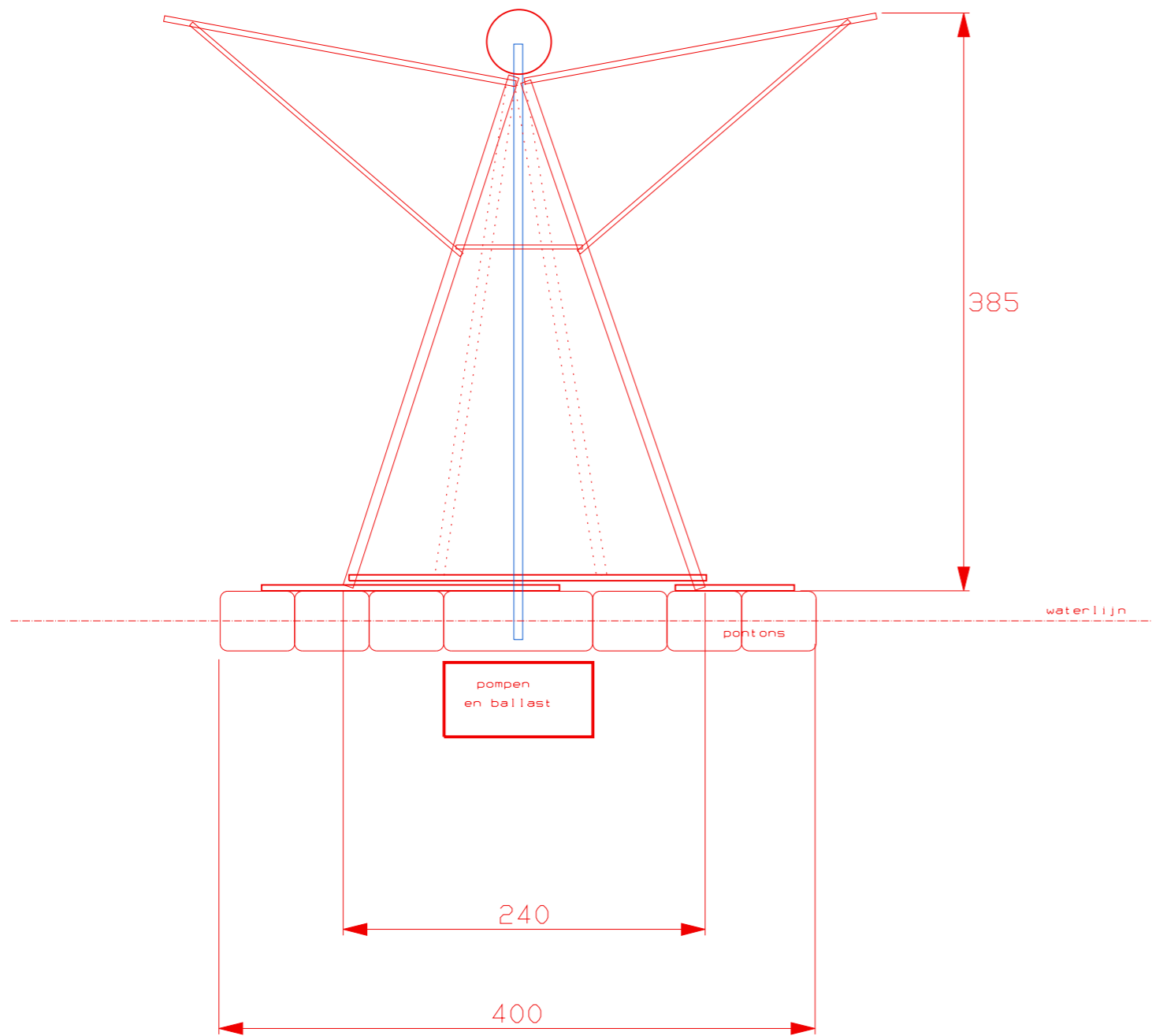
Doorsnede A - A'
